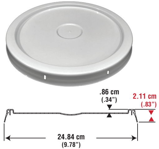
618 GASKET LID
